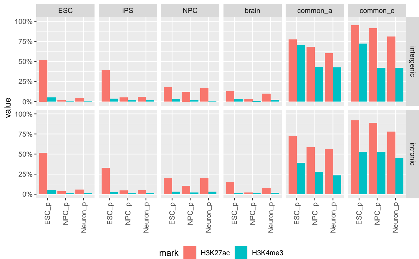
without.input.rep1_macs2
