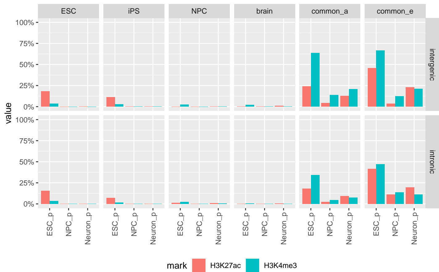
with.input.rep1_macs2
