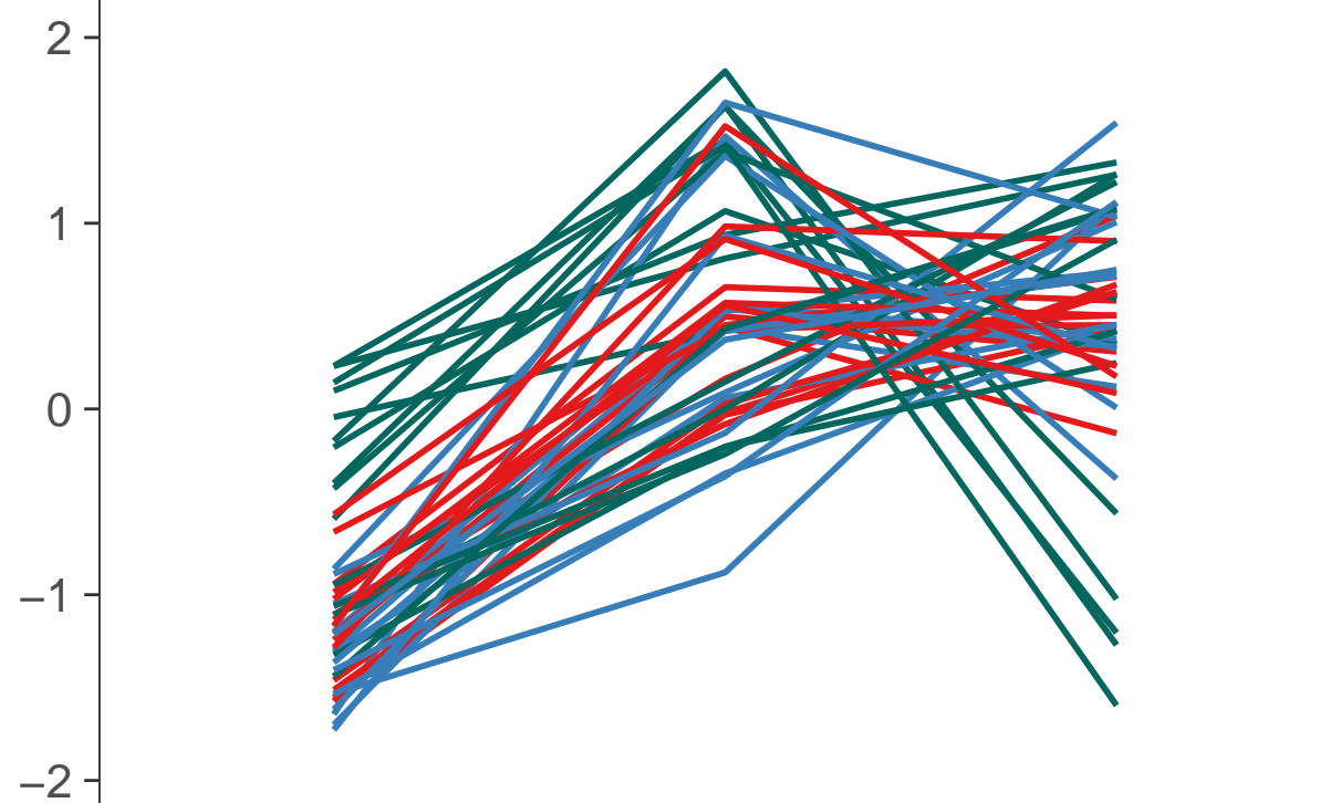
SGs_04_WP_LP_specific
