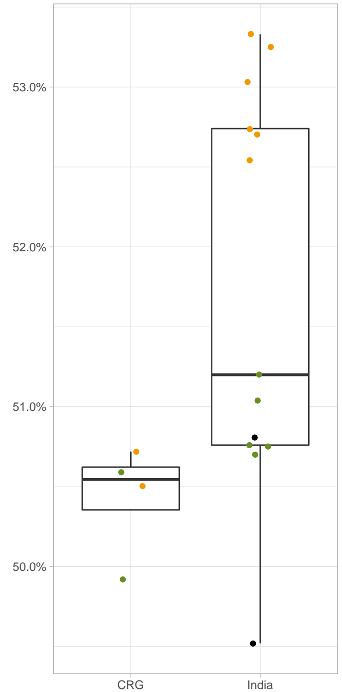
GC_Percentage
